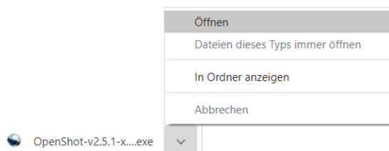
ABB.4, EXE-DATEI ÖFFNEN
