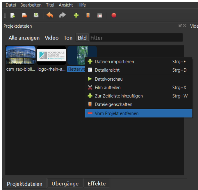
ABB. 7, KURZMENÜ
