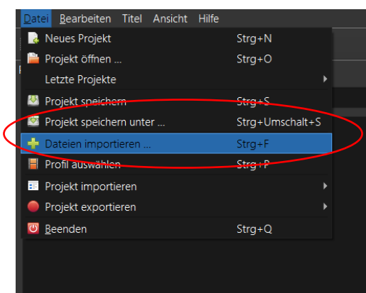
ABB.6, DATEIEN IMPORTIEREN
